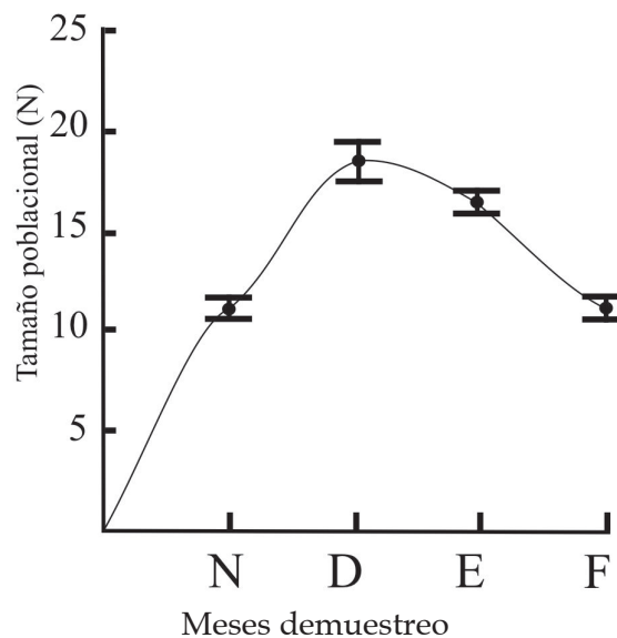
Figura 4. Fluctuación del tamaño poblacional mensual en el canal Cacalotillo, Oaxaca, México.
